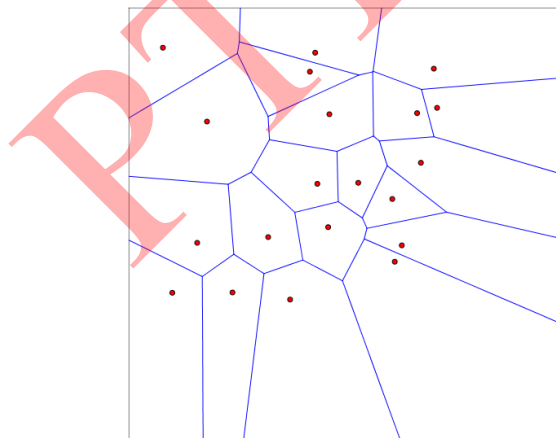
Hình 5.11. Hàm phân loại tạo ra từ thuật toán k-NN với k = 1 .
