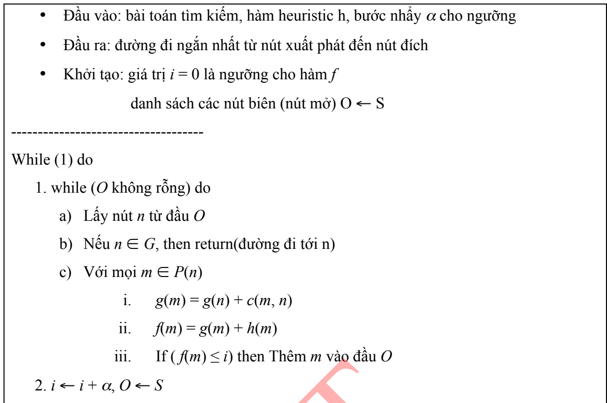
Hình 2.15. Thuật toán A* sâu dần
